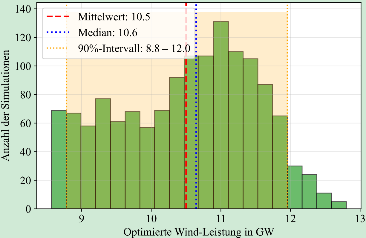
3. Unsicherheit Optimierte Wind-Leistung aus 1,400 Simulationen
