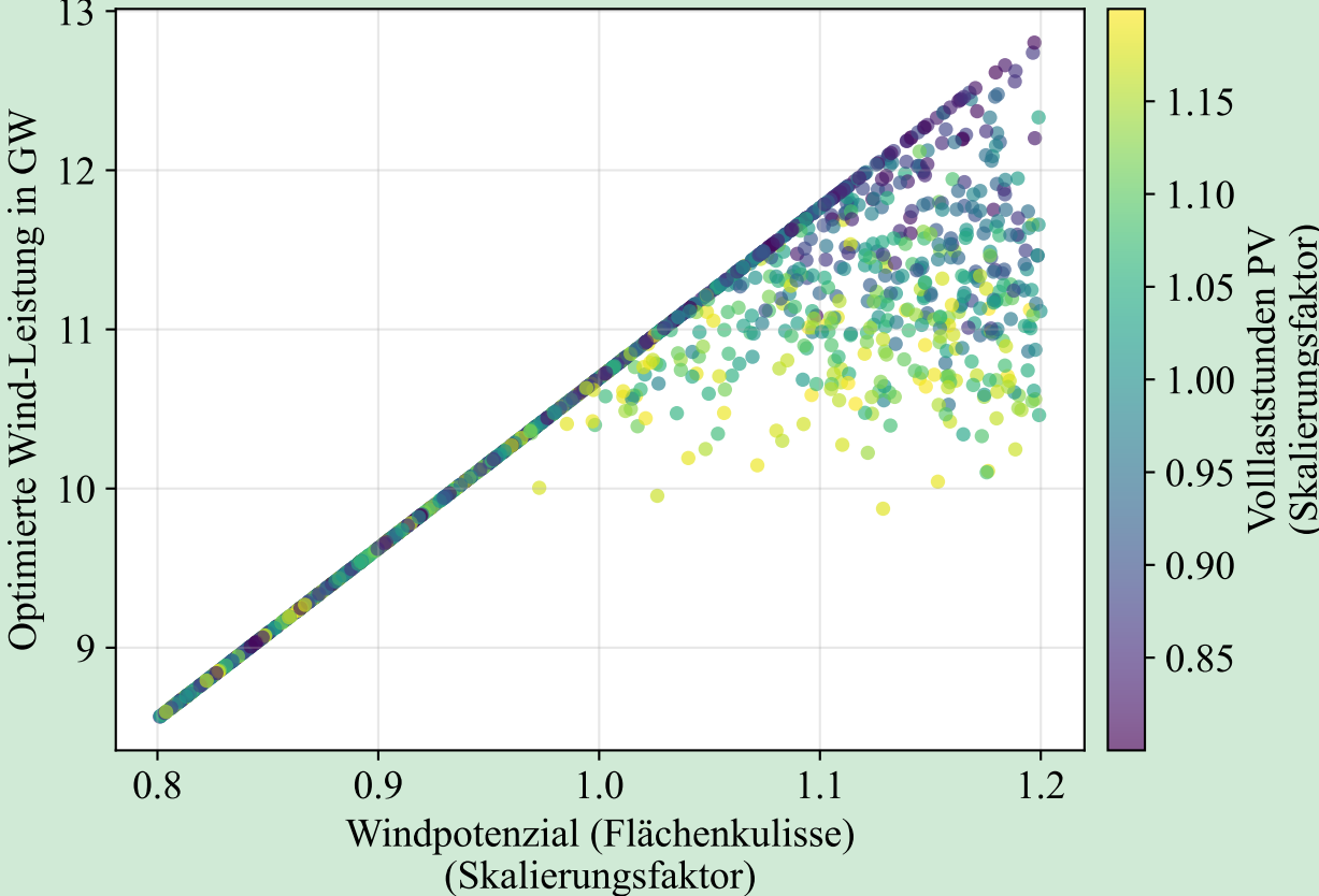
4. Parameterinteraktion Windpotenzial (Flächenkulisse) vs. Volllaststunden PV
